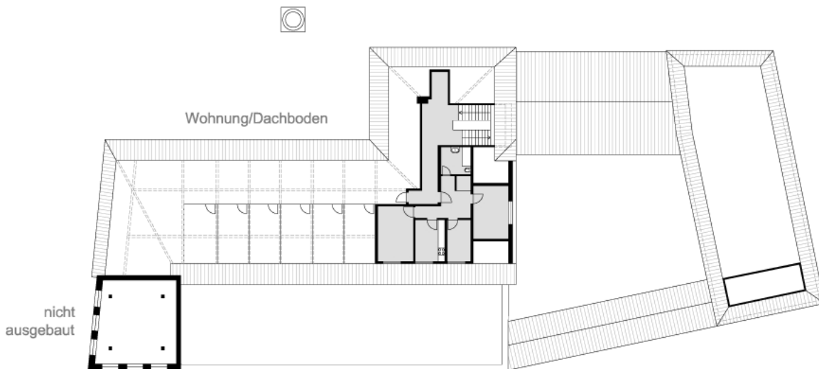
Grundriss Dachgeschoss
