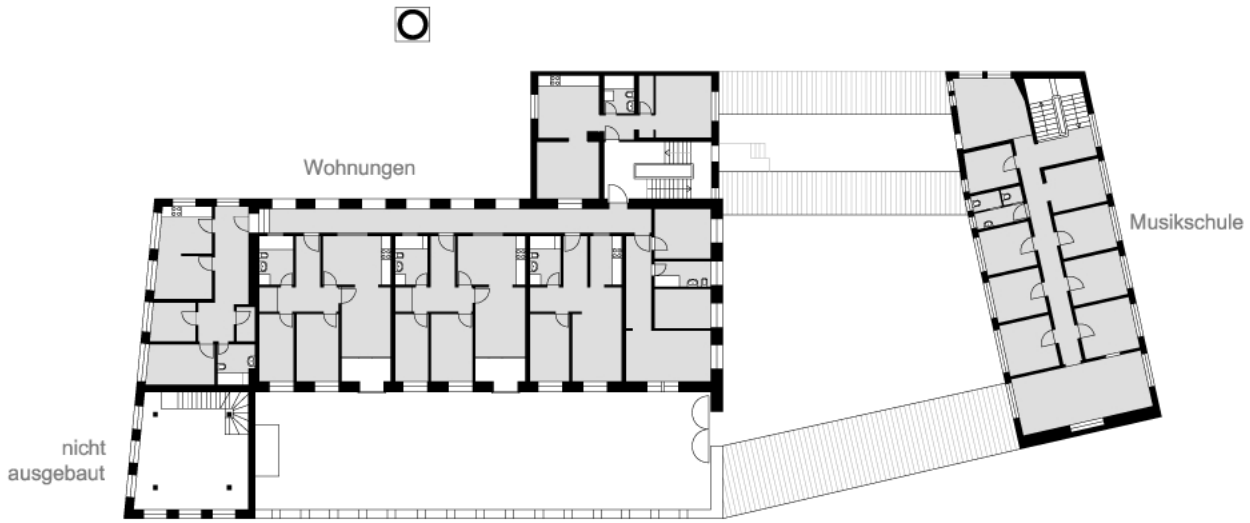
Grundriss Obergeschoss
